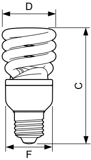
EconomyTwister 15W CDL E27 1PF/6
